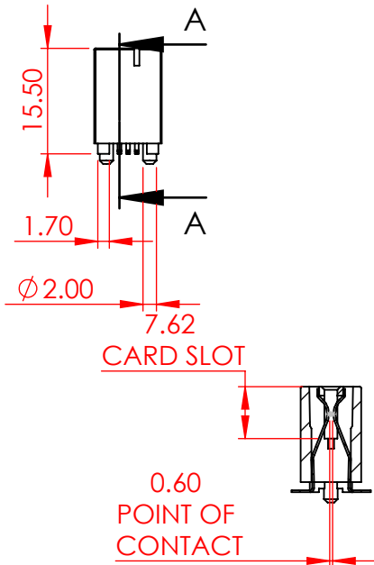
SECTION A-A SCALE 1 : 1
