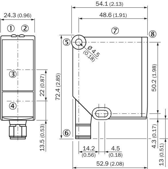
尺寸图 (尺寸单位: mm)
