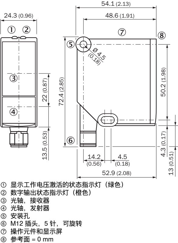
尺寸图 (尺寸单位: mm)
