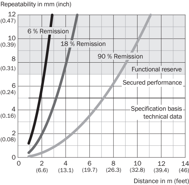
特征曲线 4) 快
