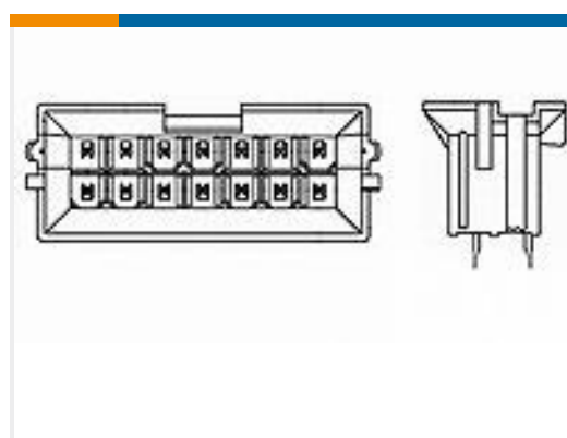
TE Part #1-1586586-2 12P VAL-U-LOK BMI VRT HDR V2
