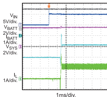
Plug in USB USB 3.0 Mode, V_{BATT} = 3.7V I_{SYS} = 2A
