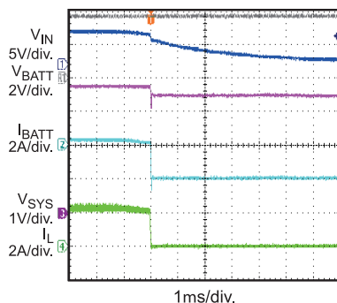
Remove Adapter V_{BATT} = 3.7V , I_{SYS} = 2A
