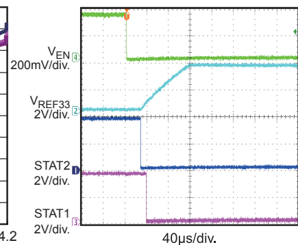
VREF Startup Waveform V_{BATT}=3.7V , En On
