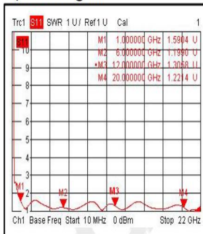
Input VSWR @+85°C
