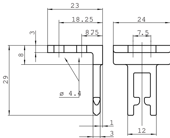
尺寸图 (尺寸单位: mm)
