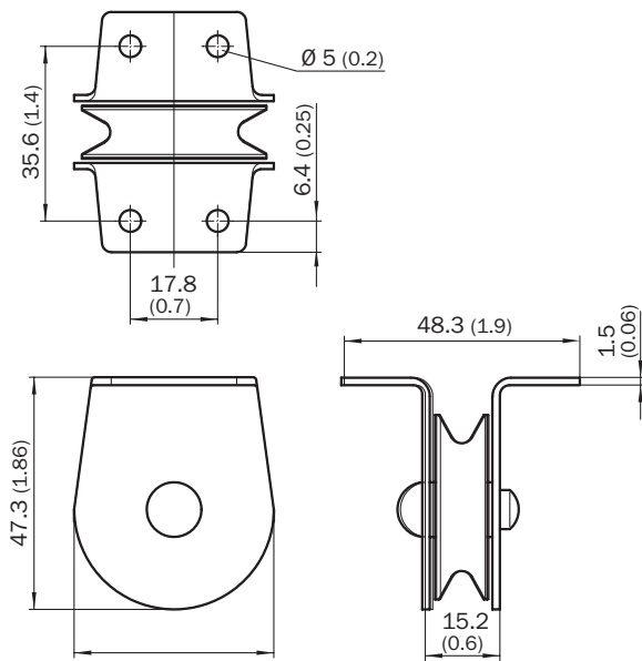
尺寸图 (尺寸单位: mm)
