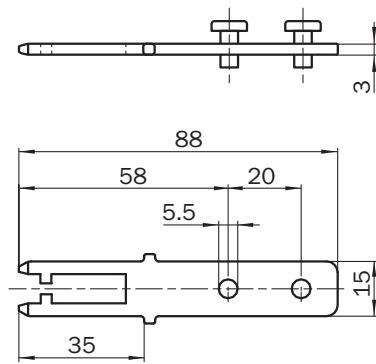
尺寸图 (尺寸单位: mm)
