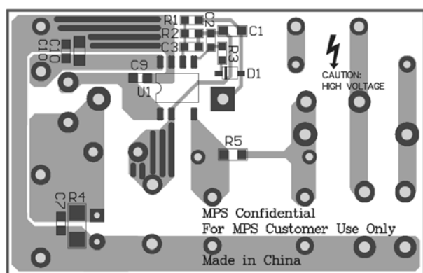
Bottom Layer
