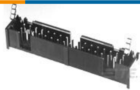
TE Part # 1-1761606-1 IDC LOW PRO HDR 34P VERT LG LAT BLK
