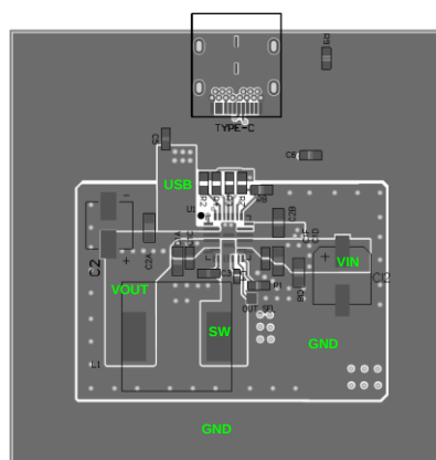
Top Layer
