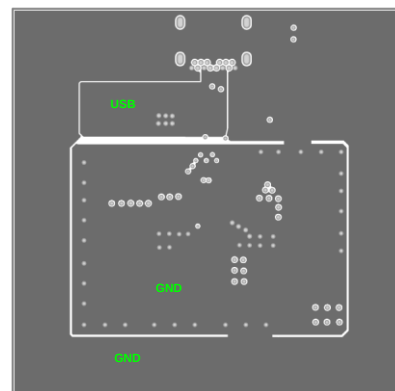
Middle Layer 1
